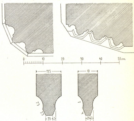
Obr. 205. Skuteč. Kostel Nanebevzetí P. Marie. Profily: 1. ostění západ. portálu, 2. ostění zazděného portálu ve věži, 3. žebra klenby v sakristii, 4. žebra klenby v kněžišti
