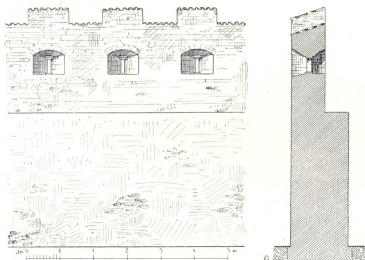
Obr. 184. Rychmburk. Hradby předhradí a řez příčný střílnou.
