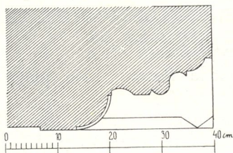
Obr. 189. Rychmburk. Zámek. Profil ostění portálu.
