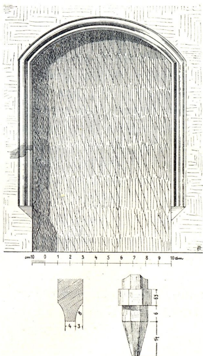
Obr. 71. Lažany. Kostel. Sedile, profil žebra a konsola v sakristií.
