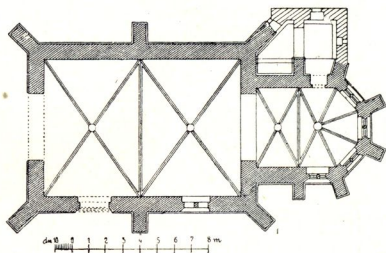
Obr. 214. Skuteč. Kostel Božího Těla. Půdorys.
