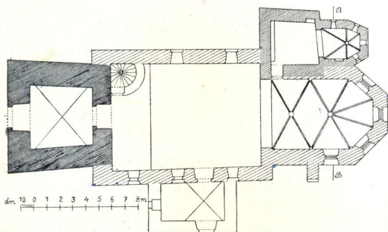
Obr. 66. Lažany. Půdorys kostela.
