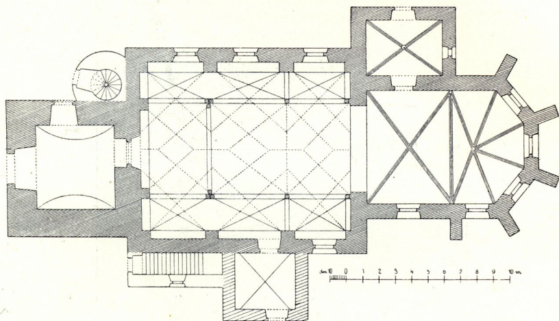
Obr. 202. Skuteč. Kostel Nanebevzetí P. Marie. Půdorys
