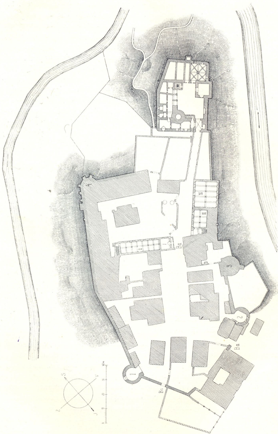
Obr. 183. Rychmburk. Přidorys hradu s předhradím. 1—4. Bašty, B a — B h Brány, I—IV. Místnosti v pivovaru a lihovaru se zachovanými klenbami.
