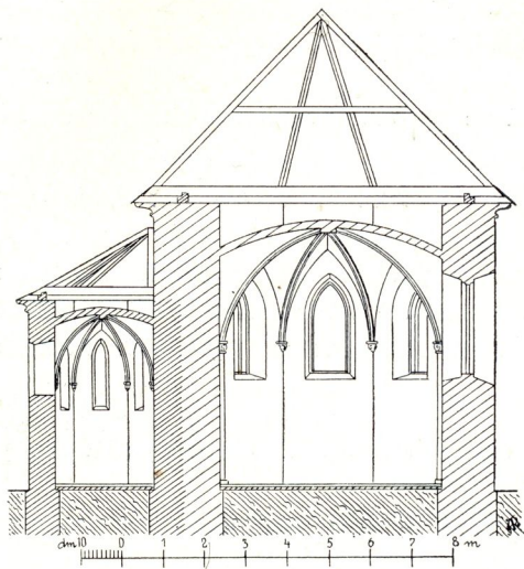
Obr. 70. Lažany. Kostel. Příčný řez kněžištěm a sakristií.
