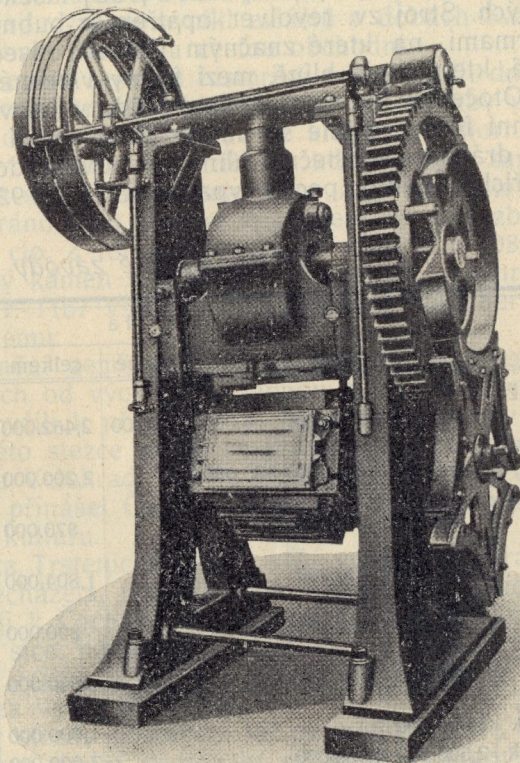
Revolverový lis na výrobu tašek.
